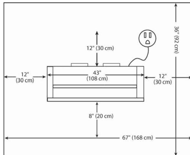
KIP 720 Draufsicht
